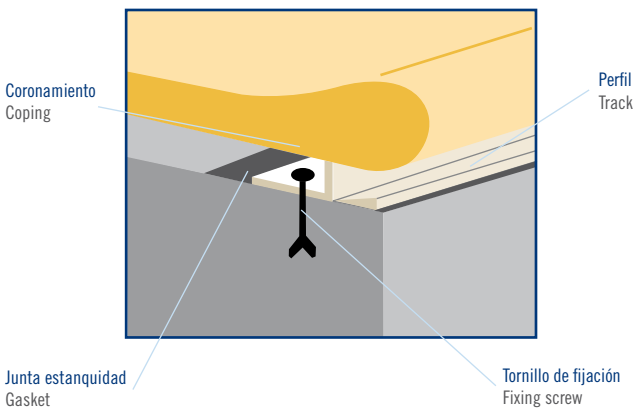
Fijación tipo “HUNG” para piscinas a construir Hung type fastening for pools to be built
