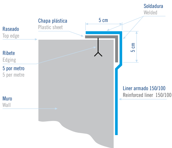
Fijación para piscinas a construir Fastening for pools under construction
