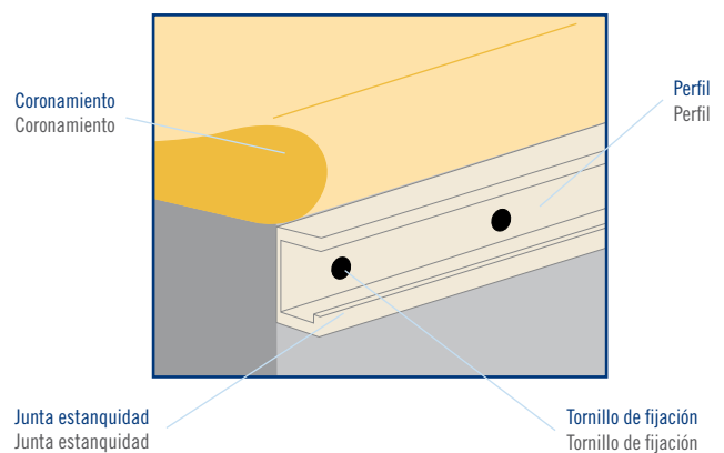
Fijación tipo “HUNG” para renovaciones Hung type fastening for renovations
