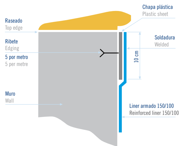
Fijación para renovaciones Fastening for renovations
